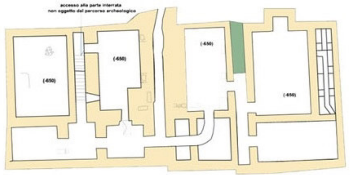
STRALCIO PIANTA A QUOTA -5.50
